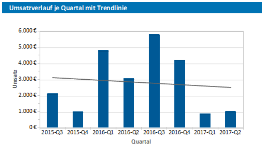
Abbildung 6.31: Ausgleichsgerade
