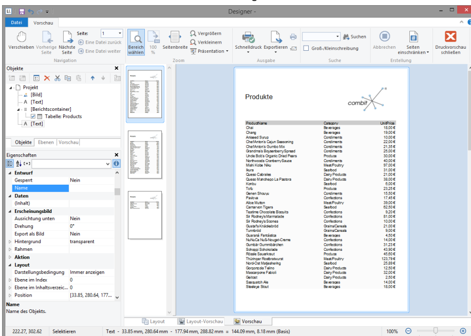
Abbildung 3.26: Echtdatenvorschau im Designer
